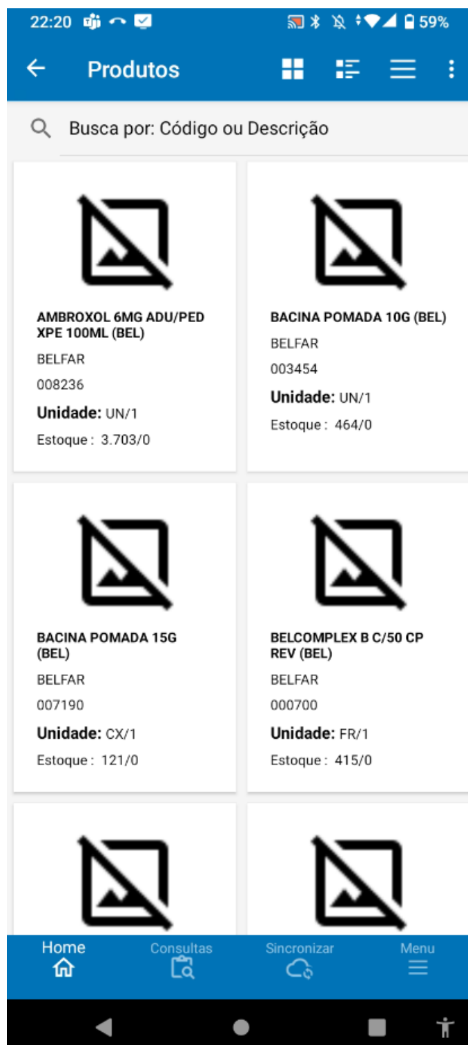
Figura 8: Tela Produtos
